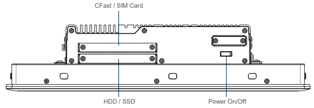
Right I/O
