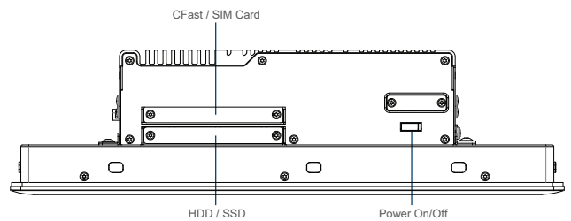
Right I/O
