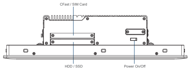
Right I/O
